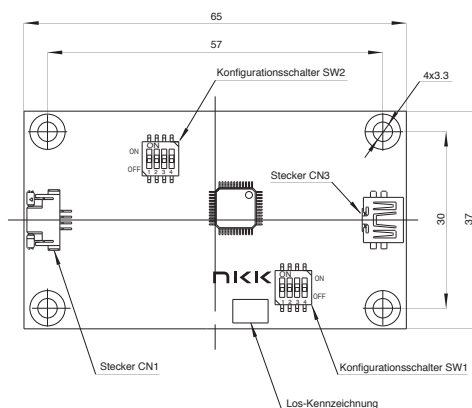
CN1 Für Anschluss eines 4-adrigen analogen Touch Screens (8 Pins)
